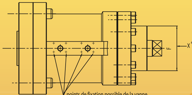
points de fixation possible de la vanne possible fixation points for the valve
